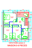
1ER ETAGE version 2 MAISON 5-6 PIECES
