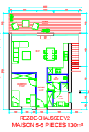
REZ-DE-CHAUSSEE v2 MAISON 5-6 PIECES 130m²
