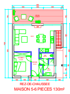
REZ-DE-CHAUSSEE MAISON 5-6 PIECES 130m²
